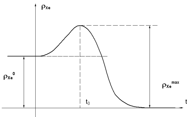
Рис. 7.2. Изменение концентрации Xe^{135} при остановке реактора
