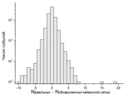
Рис. 1. Распределение разности числа обнаруженных нейронной сетью и истинным значением числа треков в событиях ДЕКОР
