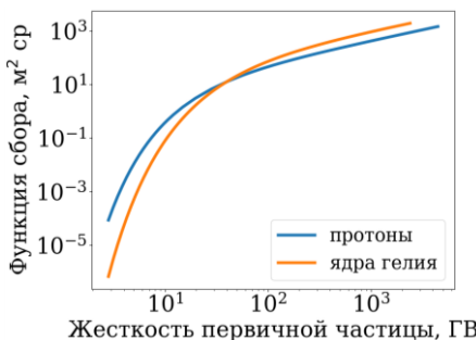
Рис.1. Функции сбора мюонного годоскопа УРАГАН
