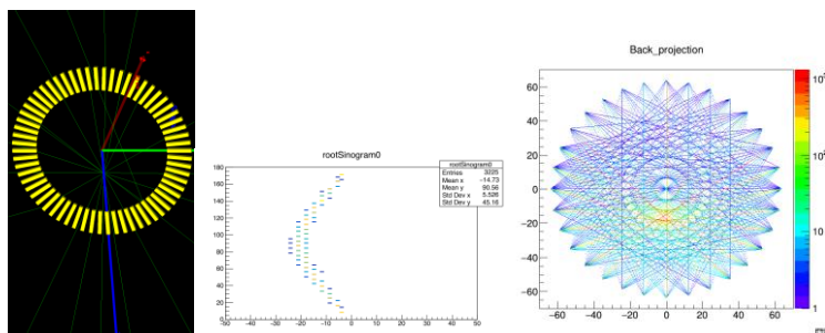
Рис.1. Получение синнограммы и обратных проекций на основе данных моделирования
