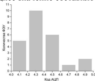
Рис. 1. Распределение значений \sigma^2/A
