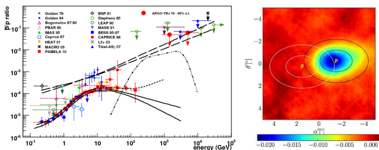
Рис.1. Слева: энергетическая зависимость отношения потоков антипротонов к протонам в ГКЛ; справа: наблюдение протонной тени по данным обсерватории HAWC, чёрный и белый эллипсы показывают предполагаемое расположение тени Луны для протонов и антипротонов.
