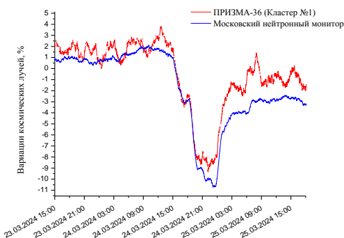
Рис. 1. Вариации космических лучей в период форбуш-понижения по данным кластера №1 установки ПРИЗМА-36 и нейтронного монитора
