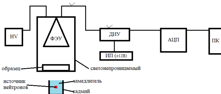
Рис. 1. Схема стенда
