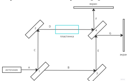
Рис.1. Классическая схема интерферометра Маха-Цендера
