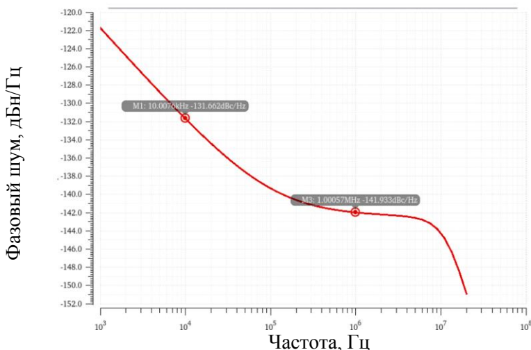
Рисунок 1 – Частотная характеристика фазовых шумов блока умножителя опорной частоты
