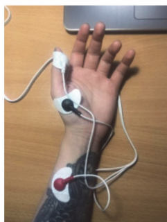
Пример считывания ЭМГ данных при жестикуляции
