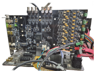
Тестовая станция для отладки SSD
