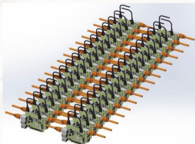
3D-модель расположения вычислительных узлов кластера
