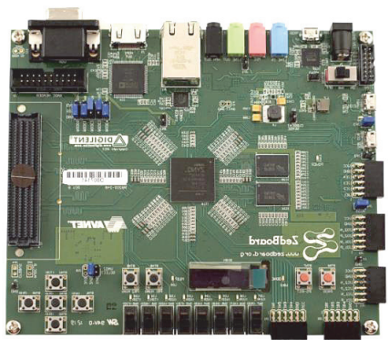
Отладочный стенд на базе системы на кристалле Xilinx Zynq 7000
