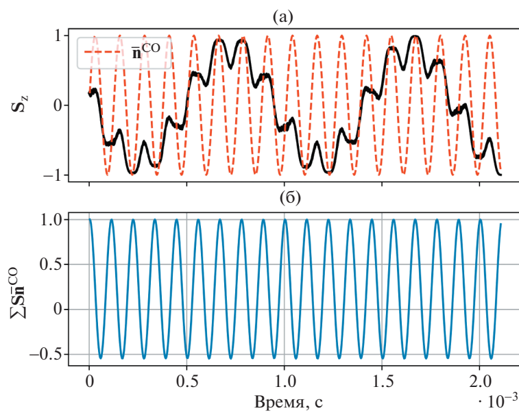
Рис. 4. Деполяризация в случае нарушения адиабатичности: \dot{\mathbf{n}} \approx 10 \cdot \Omega . (а) Эволюция ансамбля спин-векторов во времени (непрерывная линия) и оси спин-прецессии (пунктирная). (б) Поляризация пучка как функция времени. Как и ожидалось, нарушение условия адиабатичности вызывает сильные колебания величины поляризации, однако нет никаких свидетельств затухания амплитуды колебаний, а значит и декогеренции.
