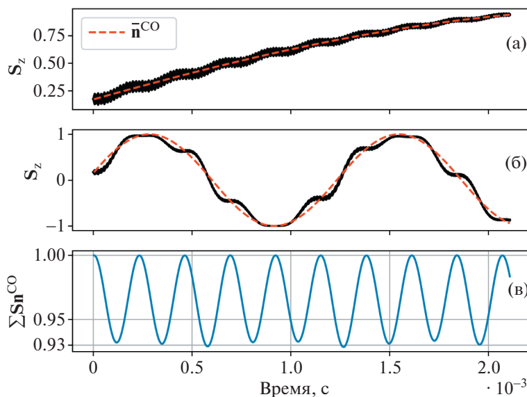
Рис. 5. Сравнение ансамбля спин-векторов и оси спин-прецессии (на замкнутой орбите) в двух других значимых случаях: \dot{\bar{n}} \approx 0.1 \cdot \Omega (адиабатический случай) (а) и \dot{\bar{n}} \approx \Omega (пограничный случай) (б). График поляризации в последнем случае (в).
