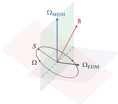
Рис. 1. Томас–БМТ спин-прецессия. (Вектор \Omega_{\text{EDM}} многократно увеличен для удобства восприятия). Вектор \vec{n} – совокупная ось спин-прецессии за счет обоих электрического и магнитного моментов.
