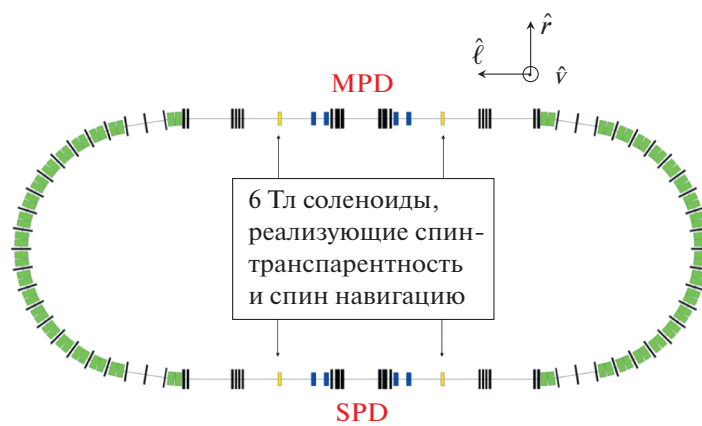
Рис. 3. Оптическая структура использованная при моделировании.
