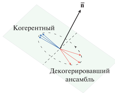
Рис. 2. Спин-декогеренция.
