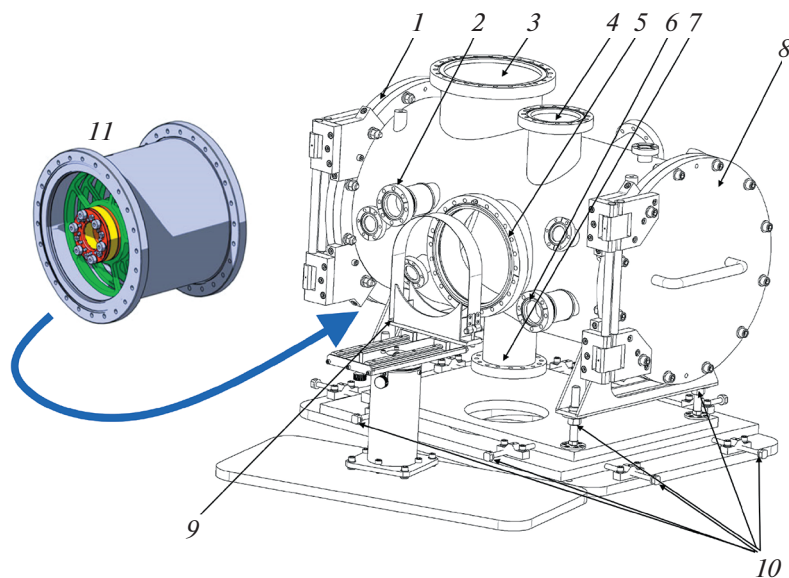
Рис. 2. Чертеж общего вида мишенной камеры со стороны блока нагрева мишени: 1 – вакуумная дверь, 2 – патрубок под вход охладителя криоэкрана, 3 – патрубок под ТМН, 4 – патрубок под цилиндр Фарадея пучка легких ионов, 5 – патрубок под мишенный блок, 6 – патрубок под выход охладителя криоэкрана, 7 – патрубок под цилиндр Фарадея пучка тяжелых ионов, 8 – вакуумная дверь, 9 – подставка под мишенный блок, 10 – средства юстировки, 11 – мишенный блок.
