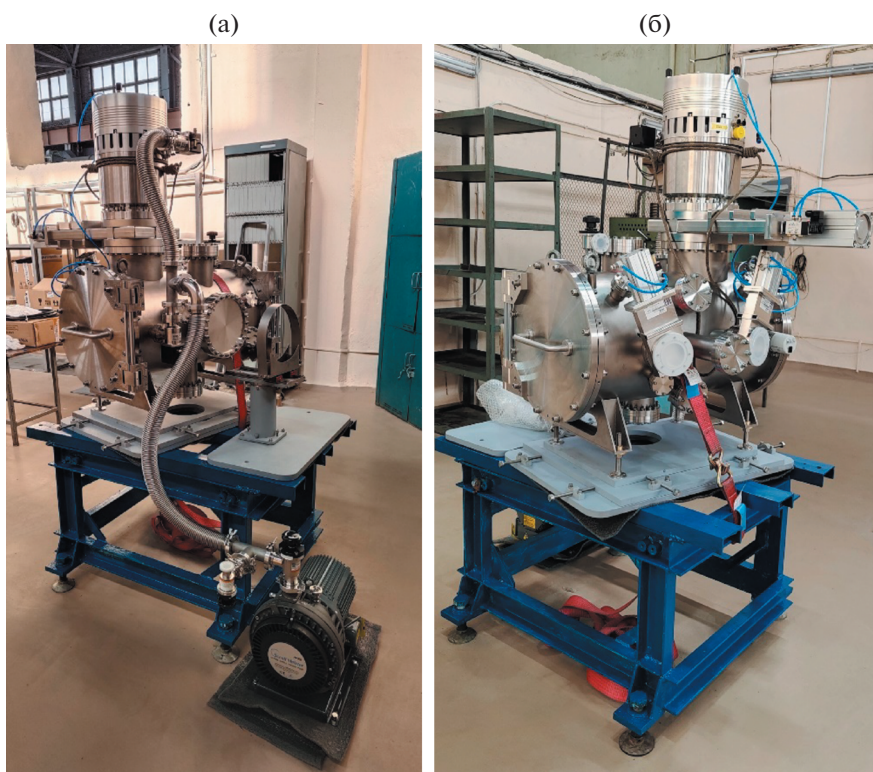
Рис. 5. Стенд испытаний вакуумной камеры: (а) вид со стороны мишенного блока, (б) вид со стороны входа пучков.
