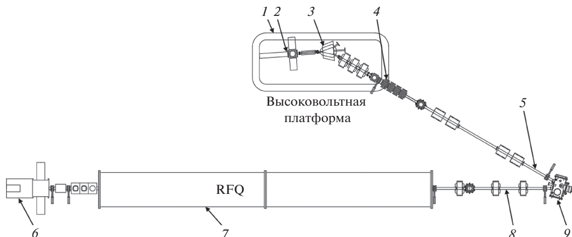
Рис. 1. Схема двухпучковой установки на базе ускорителя ТИПр-1: 1 — высоковольтная платформа, 2 — источник ионов на основе ЭЦР разряда, 3 — поворотный магнит, 4 — электростатический ускоритель, 5 — канал транспортировки легких ионов, 6 — вакуумно-дуговой источник ионов металлов, 7 — ускоряющая структура Radio-Frequency Quadrupole, 8 — канал транспортировки тяжелых ионов, 9 — мишенная камера.
