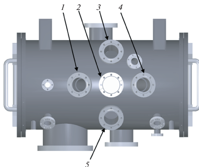
Рис. 3. Вид мишенной камеры со стороны входа пучков: 1 – вход пучка легких ионов, 2 – патрубок под устройство плазменной чистки, 3 – вакуумное окно под тепловизор, 4 – вход пучка тяжелых ионов, 5 – патрубок для ПЗС-камеры.
