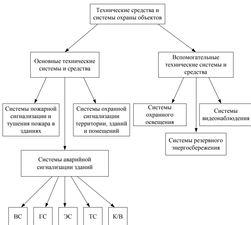
Рис. 1.4. Классификация ТСО
