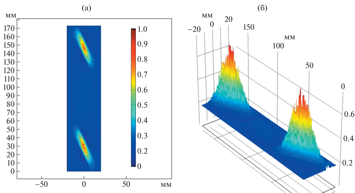
Рис. 7. Нормированное распределение индукции магнитного поля B_z на высоте 2 мм от поверхности CORC кабеля. (а) Распределение в плоскости YZ ( x = 2 мм), (б) распределение величины B_z по высоте в той же плоскости.
