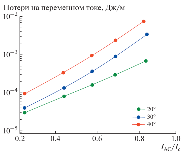
Рис. 11. Зависимость потерь на переменном токе от приложенной токовой нагрузки для различных углов намотки CORC-кабеля.
