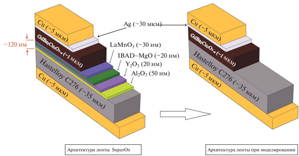
Рис. 4. Архитектура ВТСП лент фирмы SuperOx. (а) Реальная структура слоев ленты, (б) иллюстрация упрощения структуры, применяемой при моделировании.
