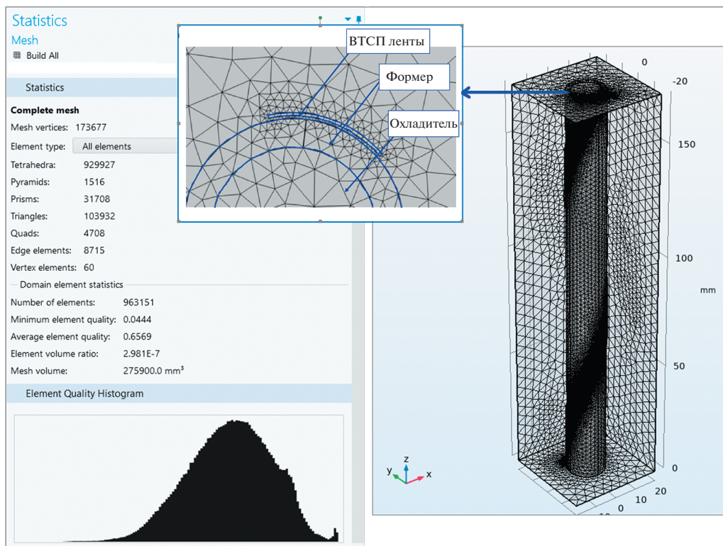
Рис. 5. Сетка модели CORC-кабеля, на вставке — увеличенный вид сверху.
