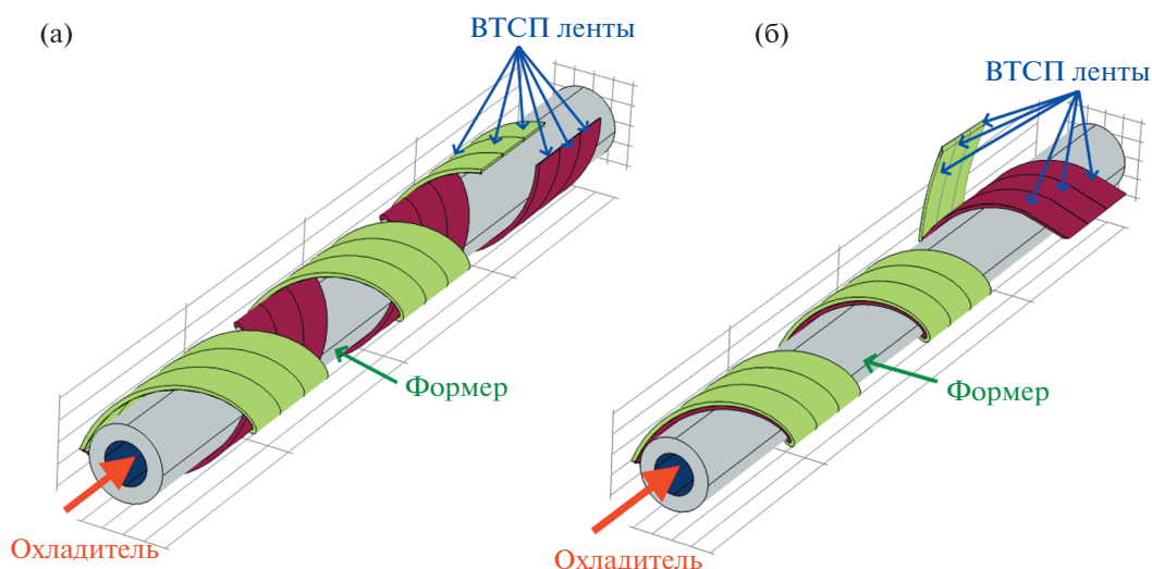
Рис. 1. Схематическое изображение конструкции многослойного CORC-кабеля: (а) конструкция кабеля со встречной намоткой ВТСП лент, (б) конструкция кабеля с параллельной намоткой ВТСП лент.
