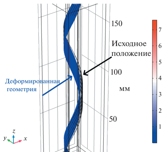
Рис. 12. Распределение механических напряжений по мизасу [Па] в CORC кабеле после пятого цикла нагрузки (scale factor = 5). Максимальные деформации, соответствующие более теплым оттенкам цветовой шкалы, характерны для тонкого ВТСП слоя, ввиду чего трудноразличимы на распределении.
