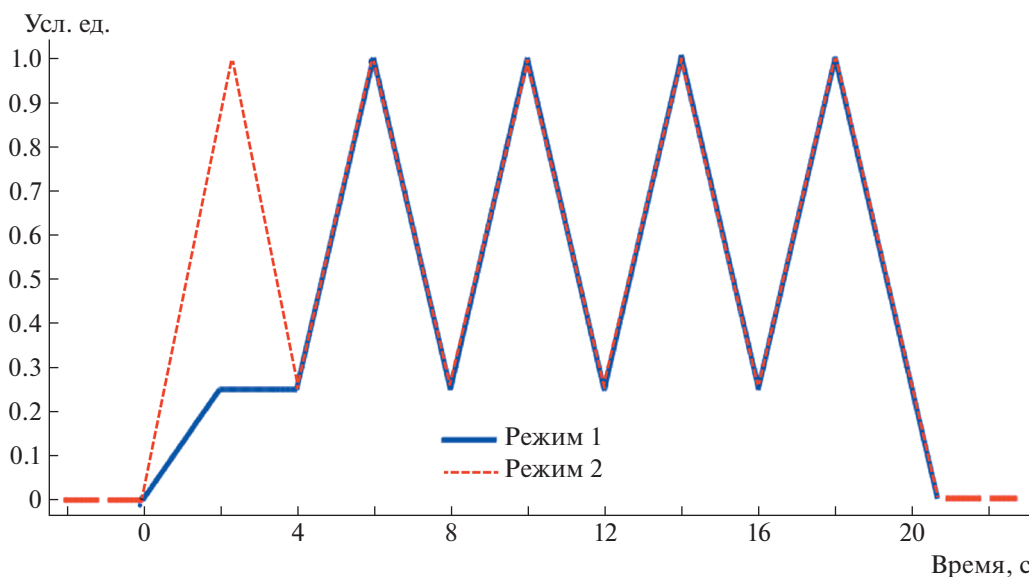
Рис. 3. Функциональная зависимость приложенной магнитной и токовой нагрузки от времени. Режим 1 — режим мягкого ввода нагрузки, Режим 2 — режим резкого ввода нагрузки.
