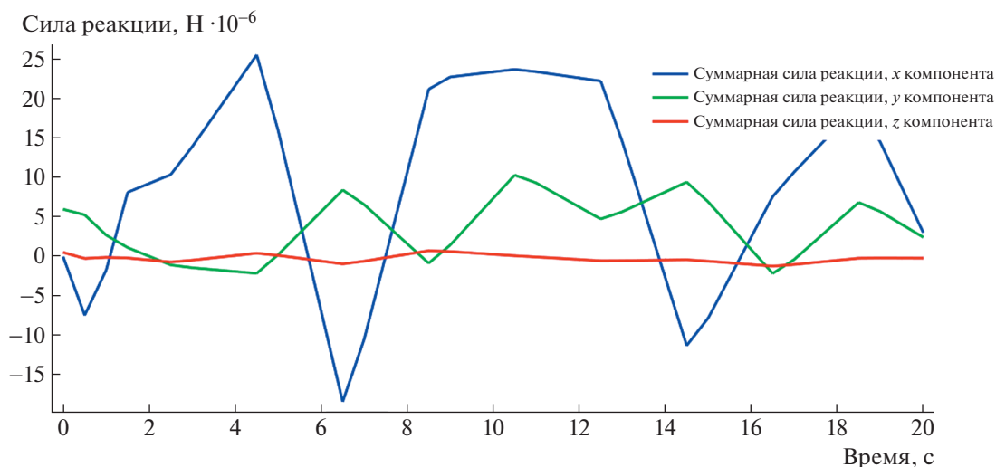
Рис. 13. Компоненты общей силы реакции опоры мельхиоровой трубки от времени для трех соседних витков CORC кабеля.
