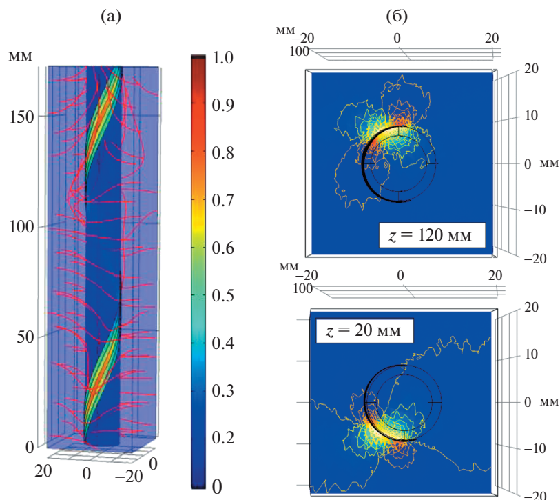
Рис. 6. Нормированное распределение магнитного поля в расчетной системе (а) и в двух плоскостях xy на различной высоте (б) в системе после ввода нагрузки в мягком режиме ( t = 2 с) (рис. 3).
