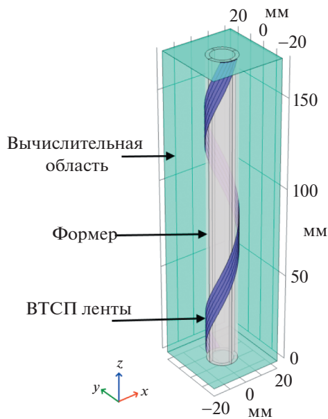
Рис. 2. Геометрия расчетной системы.
