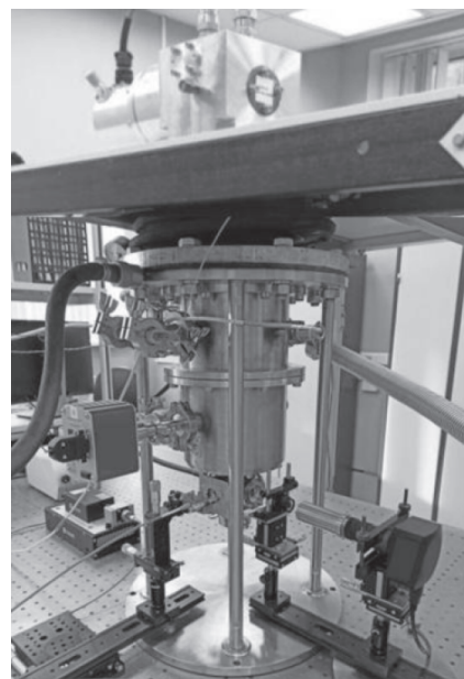
Рис. 3. Стенд для исследования мишеней при низких температурах.
