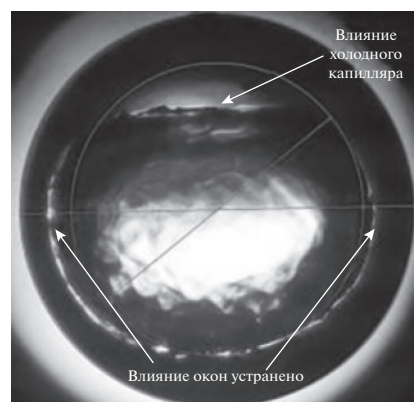
Рис. 6. Влияние холодного капилляра и теплоприток от окон бокса.
