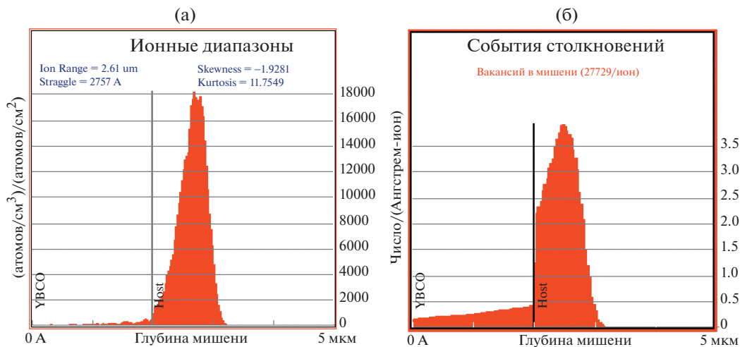
Рис. 1. Профили радиационного повреждения по толщине образца при облучении ионами \text{Cu}^+ E = 6.3 МэВ: (а) распределение ионов \text{Cu}^+ внутри образца; (б) распределение плотности вакансий внутри образца.
