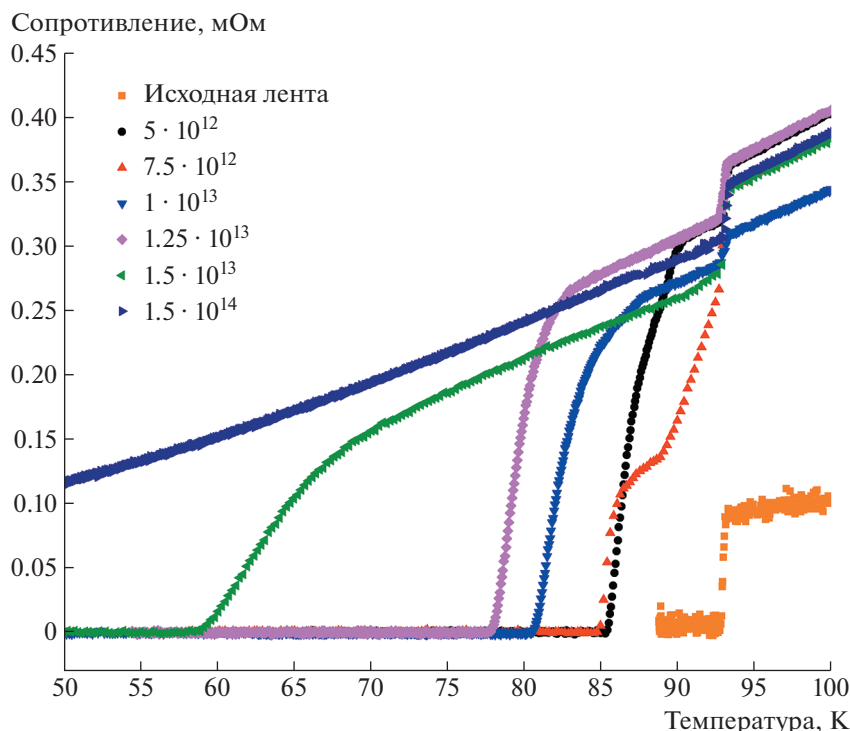
Рис. 2. Зависимости R(T) при различных флюенсах в диапазоне температур 50–100 К. Облучение ионами \text{Cu}^+ E = 6.3 МэВ.
