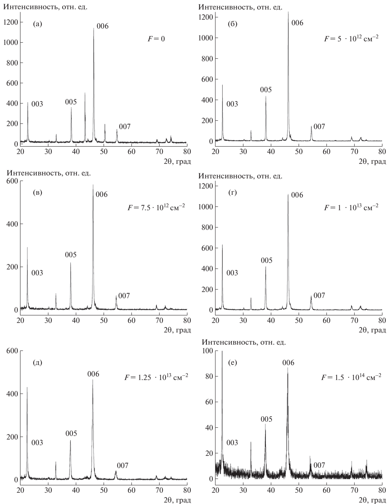
Рис. 5. Дифрактограммы исходного образца и образцов с радиационным разупорядочением. Флюенсы указаны на рисунках.
