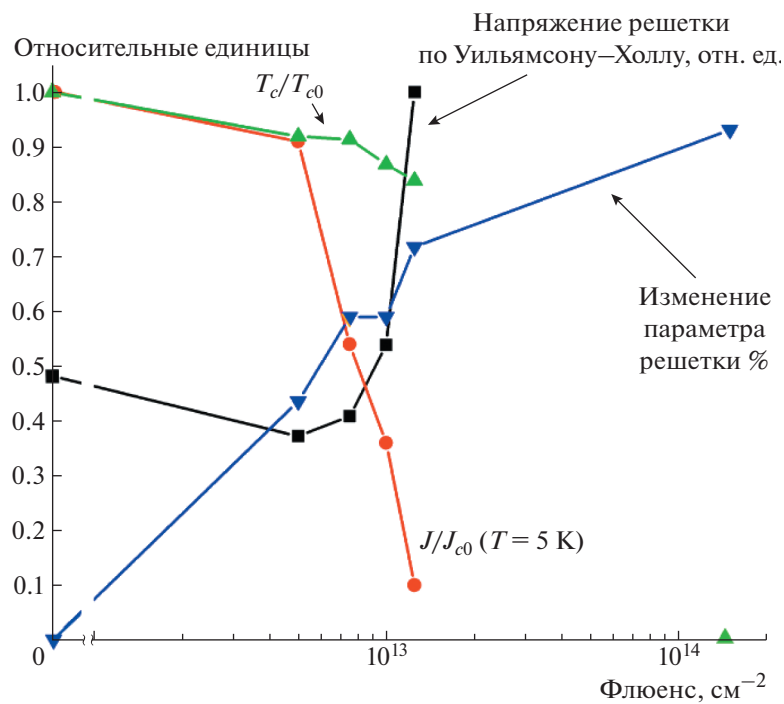
Рис. 7. Относительное изменение критической температуры — зеленые треугольники, относительное изменение критического тока — красные круги, изменение параметров решетки вдоль оси c [%] — синие треугольники и напряжение решетки по Уильямсону–Холлу [отн. ед.] — черные квадраты при увеличении флюенса облучения ионами \text{Cu}^+ .
