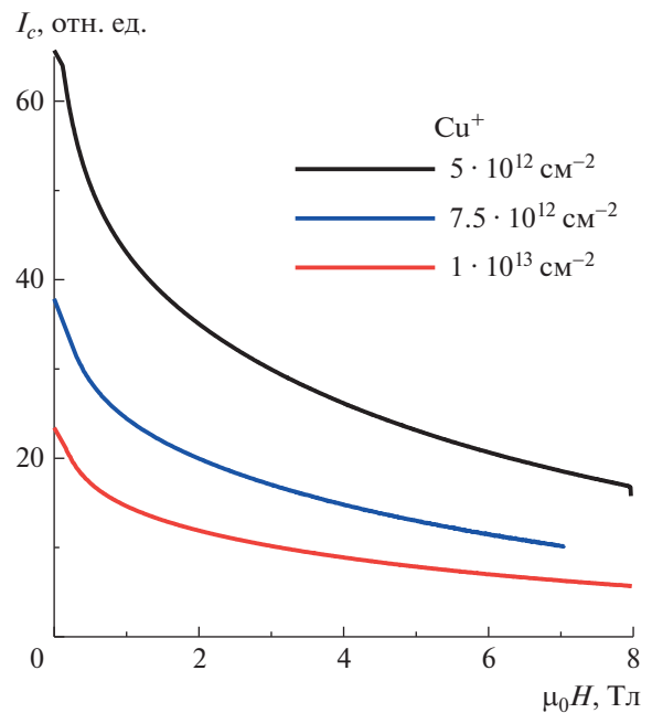
Рис. 4. Пример зависимостей критического тока от напряженности магнитного поля для различных флюенсов, T = 20 К. Облучение ионами \text{Cu}^+ E = 6.3 МэВ.
