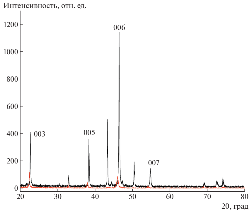
Рис. 6. Дифрактограммы исходного образца (черная кривая) и образца, облученного максимальным флюенсом 1.5 \cdot 10^{14} \text{ см}^{-2} (красная кривая)
