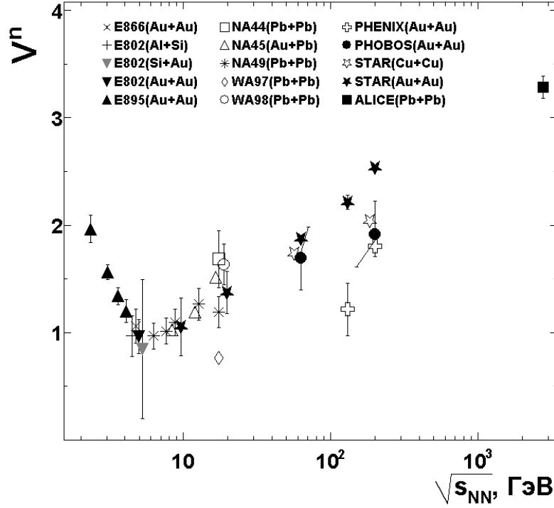
Рис. 5. Зависимость V^n(\sqrt{s_{NN}}) для различных ядро-ядерных столкновений при \langle k_\perp \rangle \simeq 0.2 ГэВ/с. Экспериментальные результаты представлены для центральных столкновений (в случае E802 для Al+Si – для событий без отбора по центральности), пар \pi^- мезонов (в случаях ALICE и STAR для (7в) – для \pi^\pm\pi^\pm пар, E802 для Al+Si – для пар \pi^+ мезонов). Показаны статистические погрешности (для NA44 – полные погрешности).
