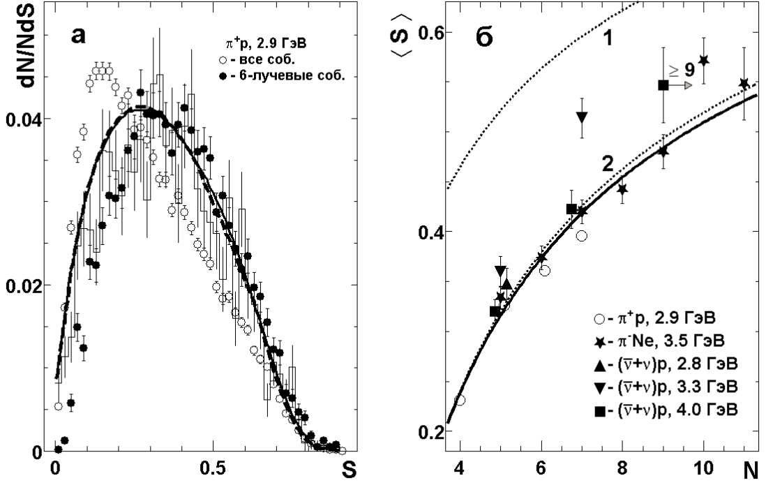
Рис. 1. Распределения по S для реакции (3\nu) и для e^+e^- аннигиляции (гистограмма) при \sqrt{s} \approx 3 ГэВ (а). Кривые – расчеты для e^+e^- по модели изотропного фазового объема (штриховая) и по модели с учетом образования струй (сплошная). Результаты и кривые для e^+e^- аннигиляции взяты из [42]. Зависимость \langle S \rangle от множественности вторичных идентифицированных частиц в событии (б). Результаты для (\bar{\nu} + \nu)p взяты из [44]. Сплошная кривая соответствует фиту результатов данной работы функцией \langle S \rangle \propto N^{-0.5} , пунктирная кривая 1 (2) – изотропному распределению вторичных частиц в фазовом пространстве для нерелятивистского (релятивистского) предела [45].
