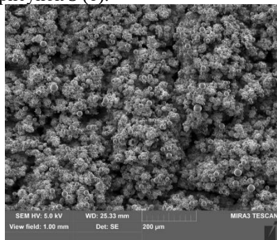
Рисунок 3. – СЭМ изображения плёнки в области пятна, (а) – увеличение 632, детектор SE, (б) – увеличение 5926, детектор BSE
