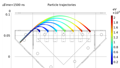
Рисунок 3. Трасектории движения протонов с различными энергиями в электрическом поле анализатора нейтралов при потенциале на верхней обкладке 1200 В. Расчёт в Comsol Multiphysics 5.6.
