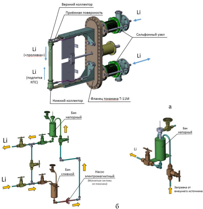
Рисунок 1 – 3D-модель лимитера литиевого квазистационарного типа токамака T-11M: а – лимитер; б – внешняя система подпитки для организации замкнутого контура циркуляции лития; в – внешняя система подпитки для подпитки одного из коллекторов
