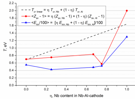
Рис. 3 Оценки критической температуры сплавов Nb-Al из среднего заряда ионизованной плазмы и их кинетической энергии с усреднением по доли компонент
