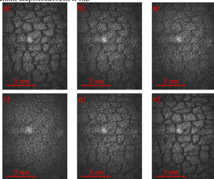
Рис. 1 – Снимки поверхности образца при облучении после растрескивания, полученные в разные моменты времени теплового удара. а) 85–105 мкс, б) 285–305 мкс, в) 385–405 мкс, г) 680–700, д) 880–900 мкс, е) 1580–1600 мкс.
