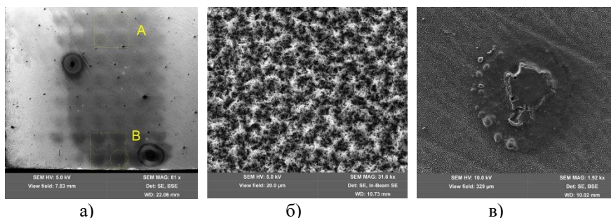
Рис. а) фото поверхности вольфрама после комплексного воздействия плазмы и электронного пучка, б) фото наноструктуры типа пух в области воздействия пучка, в) область попадания примеси на поверхность
