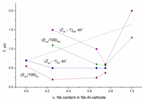
Рис. 2. Оценки критической температуры сплавов Nb-Al из среднего заряда ионов плазмы и их кинетической энергии Учет усреднение в соответствии с соотношением компонент ( \eta – доля
