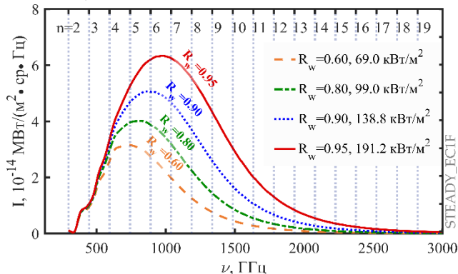
Рис. 2. Спектральные интенсивности ЭЦ излучения для ЭЦ гармоник n \geq 3 , рассчитанные кодом CYNEQ, для различных коэффициентов отражения ЭЦ волны от стенки камеры, R_w , для 4-го сценария в Таблице 1. В легенде указана интегральная по спектру мощность ЭЦ излучения на первую стенку, деленная на площадь стенки вакуумной камеры S = 876 \text{ м}^2 .
