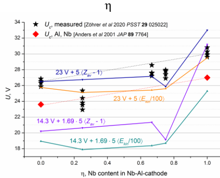
Рис. 4. Измеренные величины катодного падения U_c для сплавов Nb-Al из [4] и из [5], и оценки по среднему заряду и кинетической энергии ионизованной плазмы
