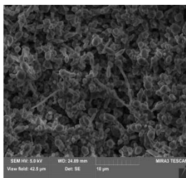
Рисунок 82 – СЭМ- изображения поверхности в зоне воздействия мощных лазерных нагрузок. (а) – увеличение 223, (б) – увеличение 14854, (в) – увеличение 15319
