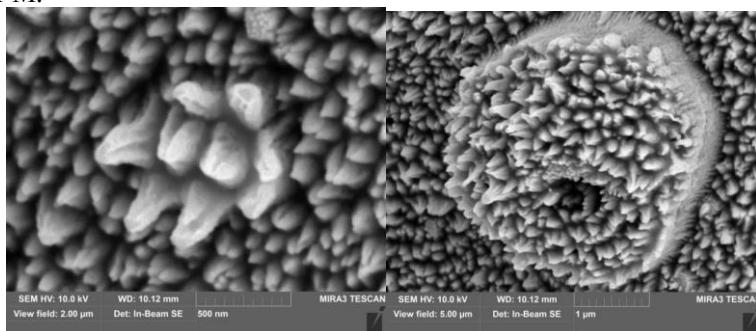
Рисунок 3 — СЭМ микрофотографии поверхности железного образца, облученного в стационарном гелиевом разряде установки ПЛМ-М
